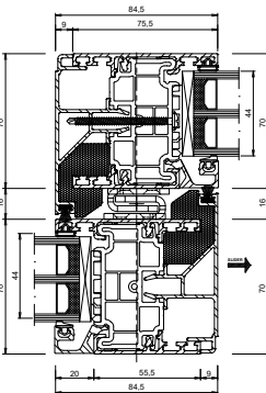
Interlock
