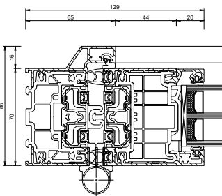
Jamb
