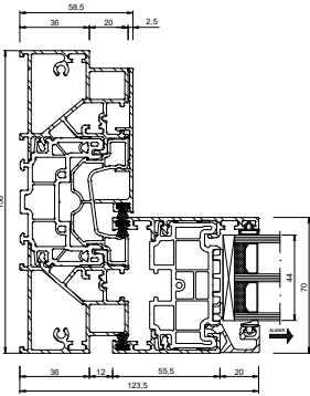
Jamb
